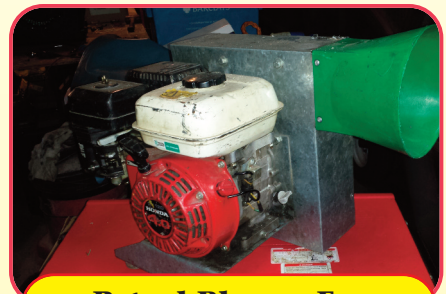
Petrol Blower Fan
